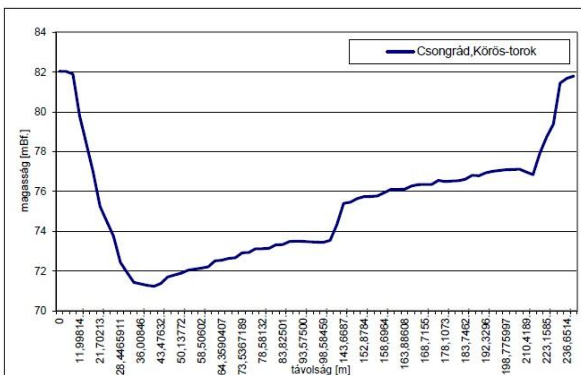
Keresztaszelvény profil ábra
